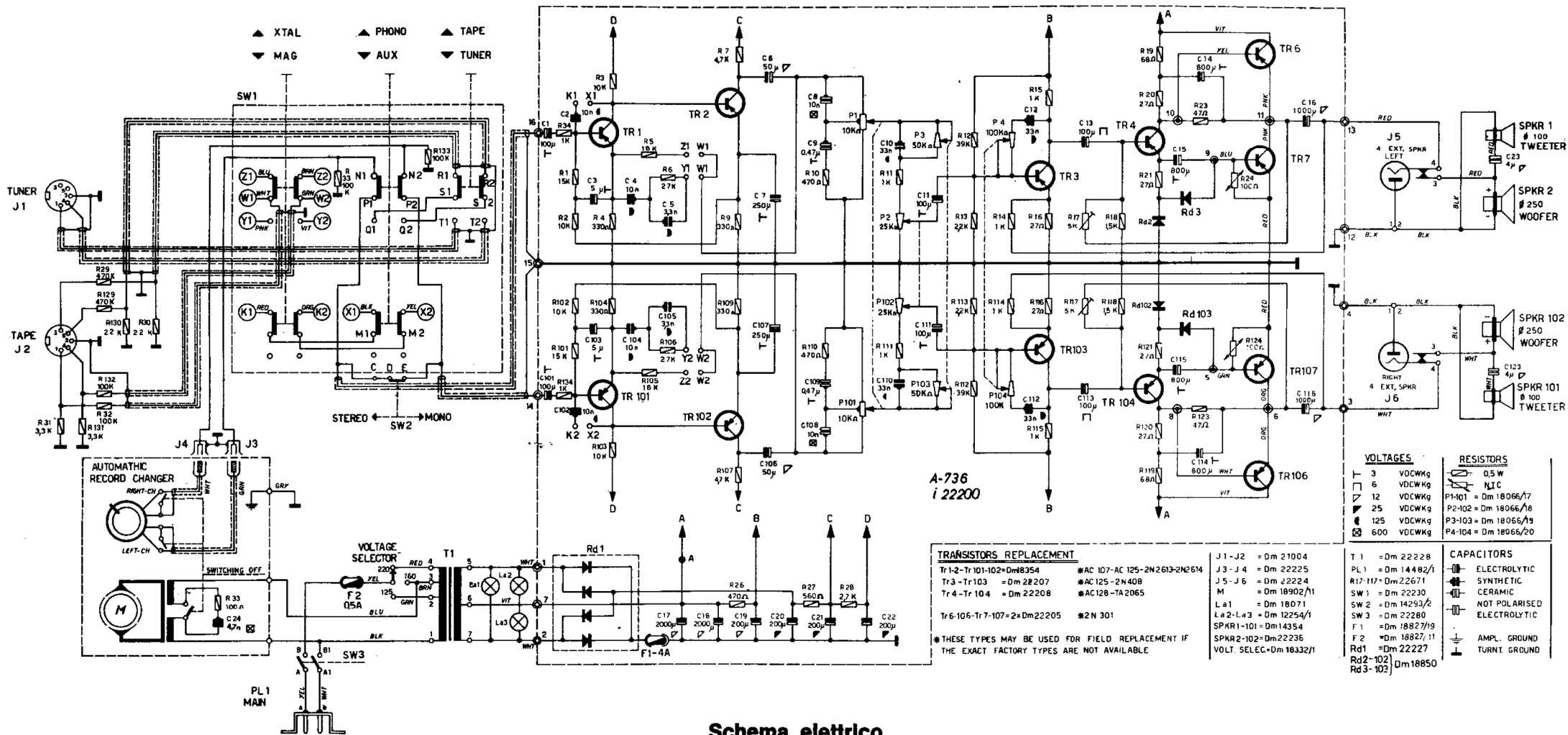
Schema elettrico
